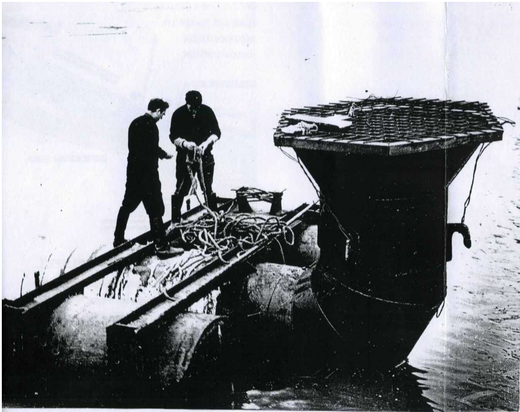
Строительство нового водозабора на станции „Заря“. г. Омск 1974г.
